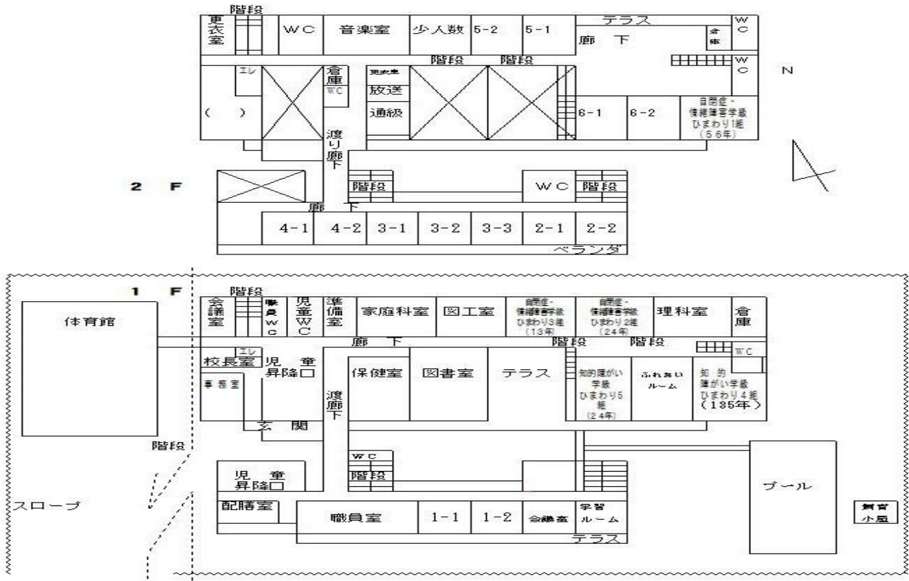
令和6年度 万田小学校 校舎平面図
